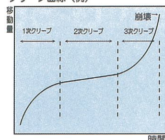
クリープ曲線 (例)
